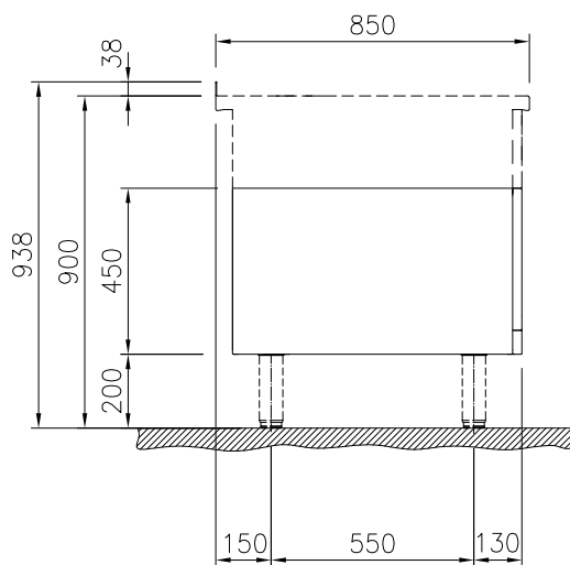
Zij aanzicht
